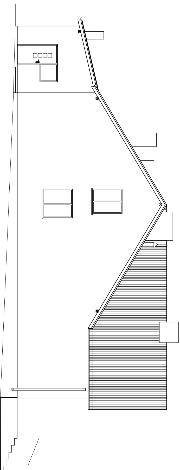
ELEWACJA WSCHODNIA
