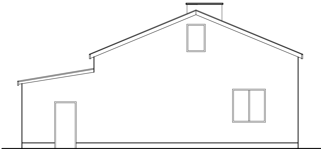
Elewacja Zachodnia
